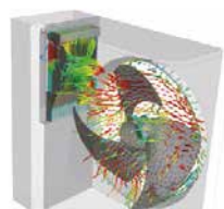
Symulacja przepływu powietrza
